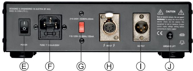
Figura 2: Mandos, entradas y salidas en la parte trasera de la unidad de control remoto
