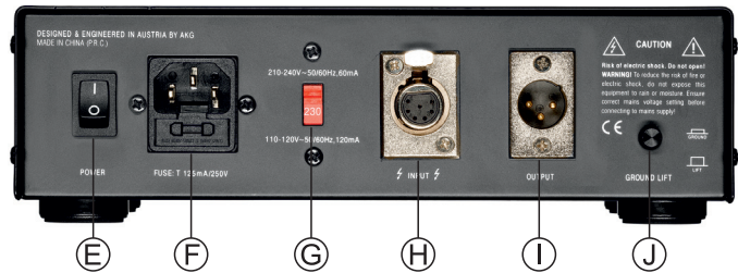
Figure 2: Commandes, entrées, sorties sur la face arrière de l'unité de commande à distance
