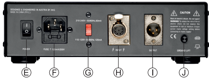
Abbildung 2: Bedienelemente, Eingänge und Ausgänge auf der Rückseite der Fernsteuereinheit
