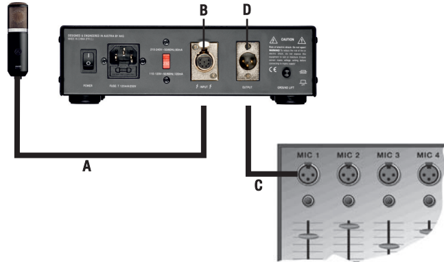
Figura 3: Conexión del micrófono a la unidad de control remoto y a la mesa de mezclas
